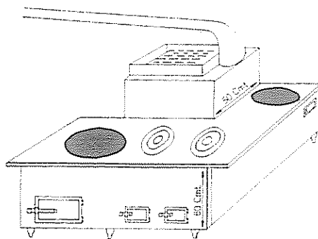
2a ábra. Kombinált gőzfejlesztő készülék [34]
