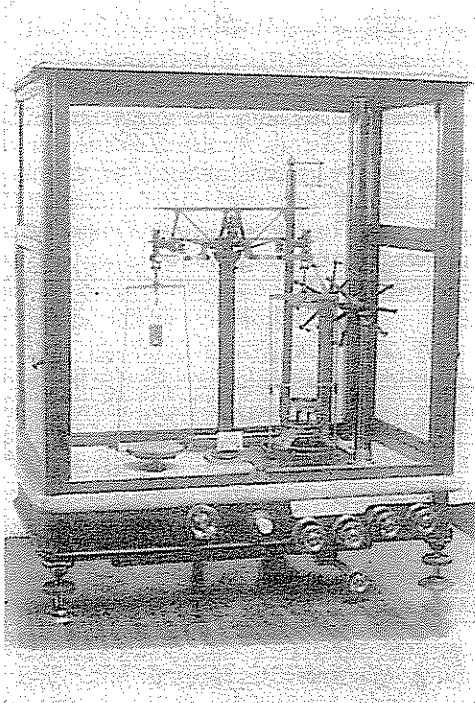
4. ábra. Nemitz-féle analitikai mérleg
