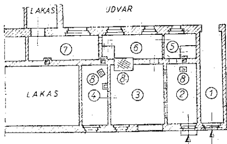
3. ábra A sümegi gyógyszer-tár alaprajza
