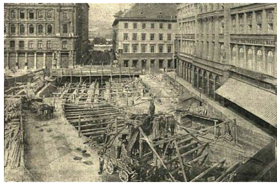
A millenniumi földalatti vasút építése
